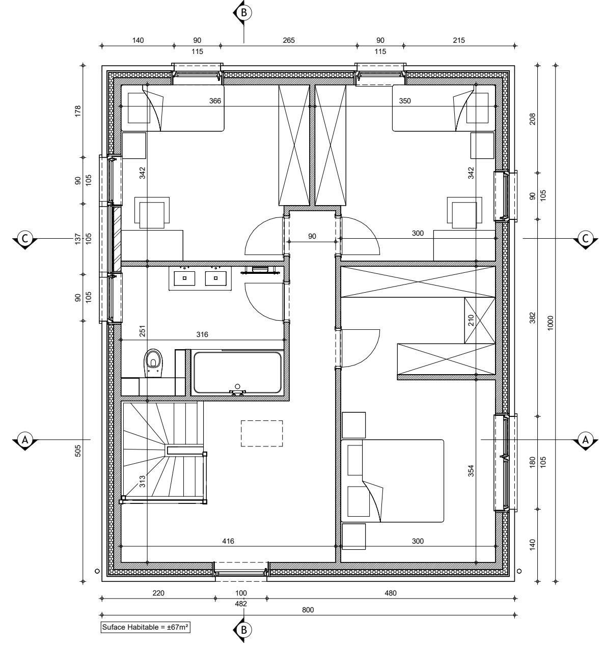
ETAGE
