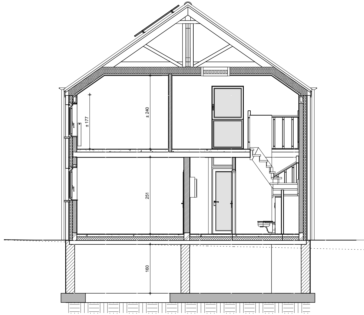
COUPE AA
