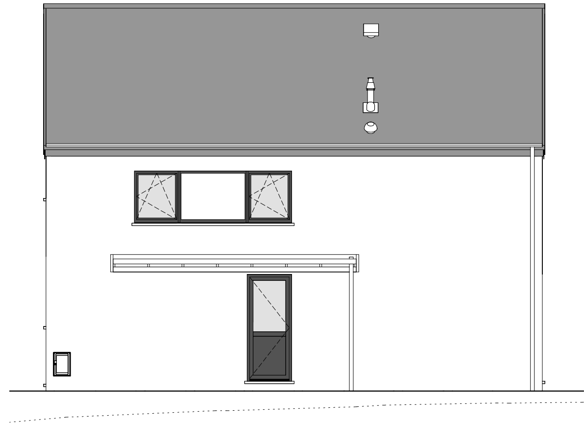
FACADE LATERALE GAUCHE
