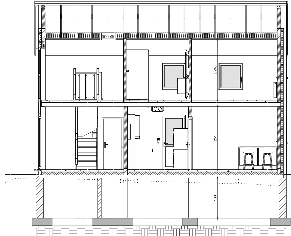
COUPE BB
