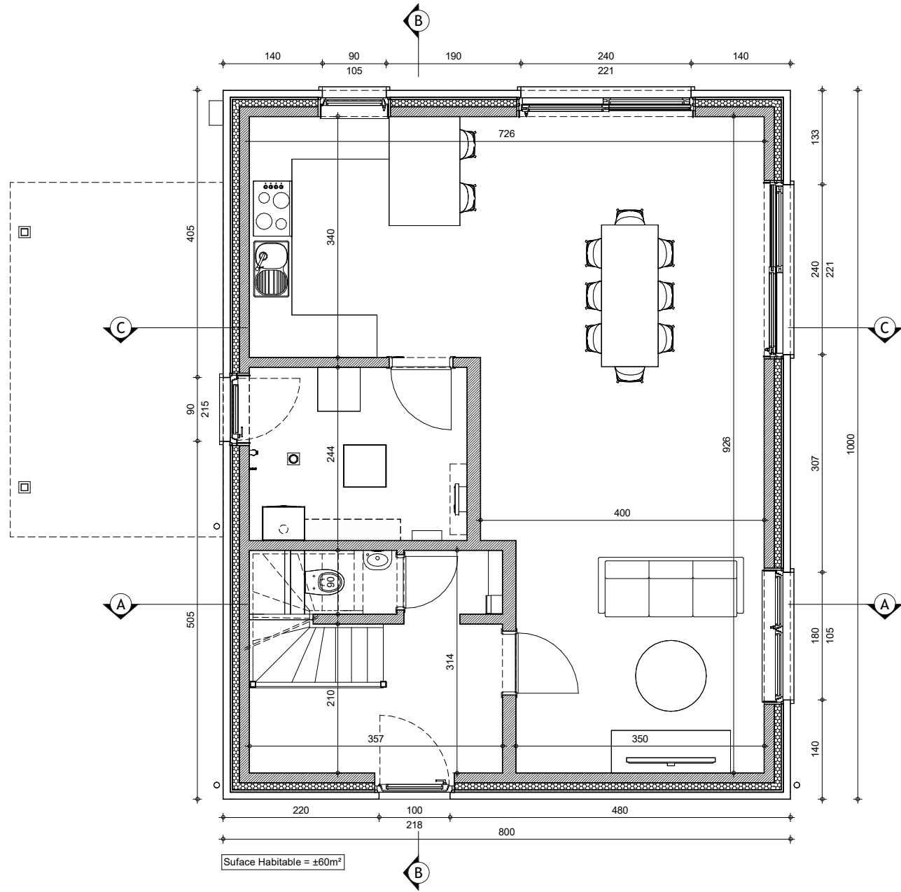
REZ-DE-CHAUSSEE
