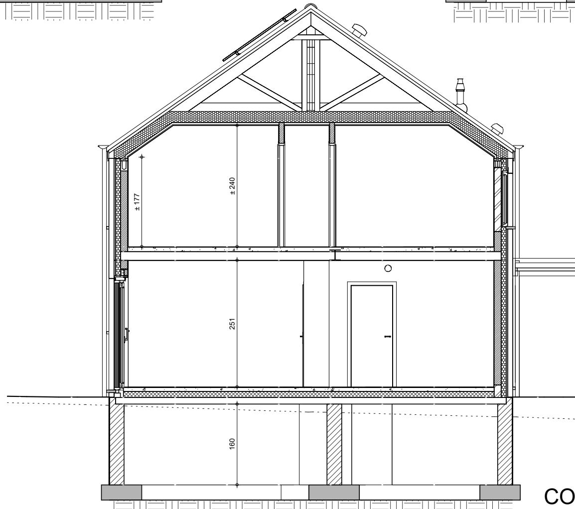
COUPE AA
